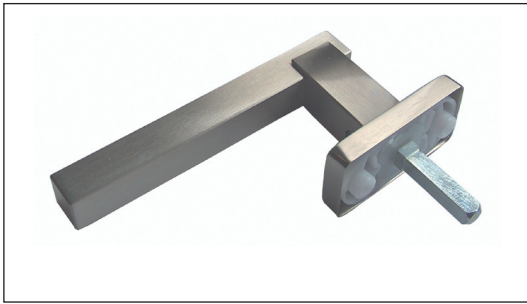
895 CW/325 ΠΟΜΟΛΟ ΜΙΚΡΟ Europa SMALL LEVER HANDLE Europa
