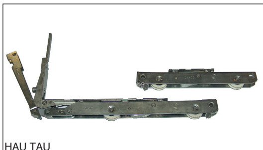
HAU TAU 193720 ΑΝΑΣΗΚΟΥΜΕΝΟ ΡΑΟΥΛΟ ΦΥΛΛΟΥ ΤΖΑΜΙΟΥ LIFT & SLIDE ROLLER FOR GLASS SASH
