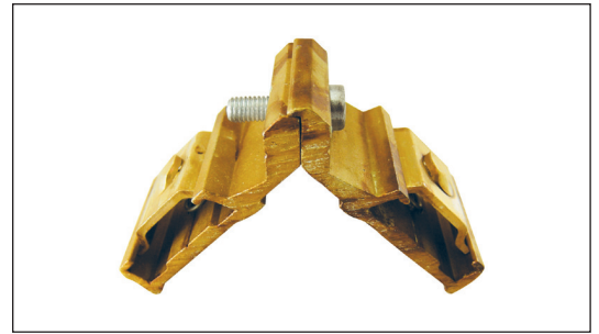
PS-11 ΓΩΝΙΑ ΣΥΝΔΕΣΕΩΣ ΦΥΛΛΟΥ ΠΑΤΖΟΥΡΙΟΥ ΚΑΙ ΟΔΗΓΩΝ CORNER JOINT FOR SHUTTER SASH & DRIVERS
